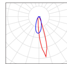
ASYM. 20°x40°
