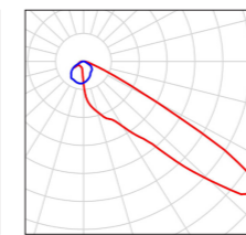
ASYM. 22°x50°
