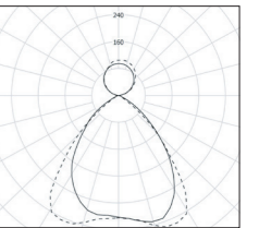
UGR19 louvre
