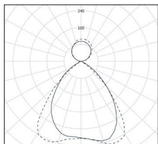
UGR19 louvre
