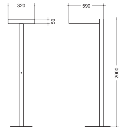
Technische Skizzen | Technical sketches
